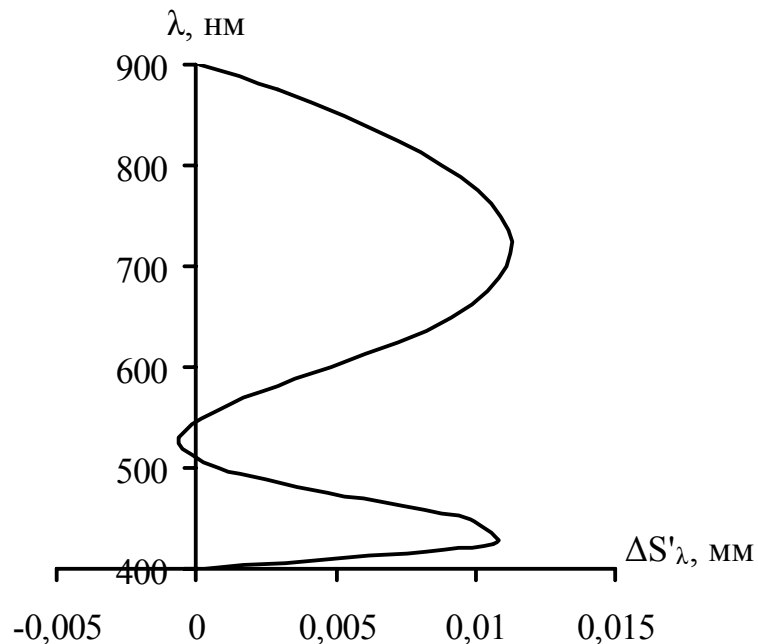
Рис.4 Остаточный хроматизм системы с f'=1000 мм, выполненной из стекол ОК1 – СТК19 – ТΦ12
