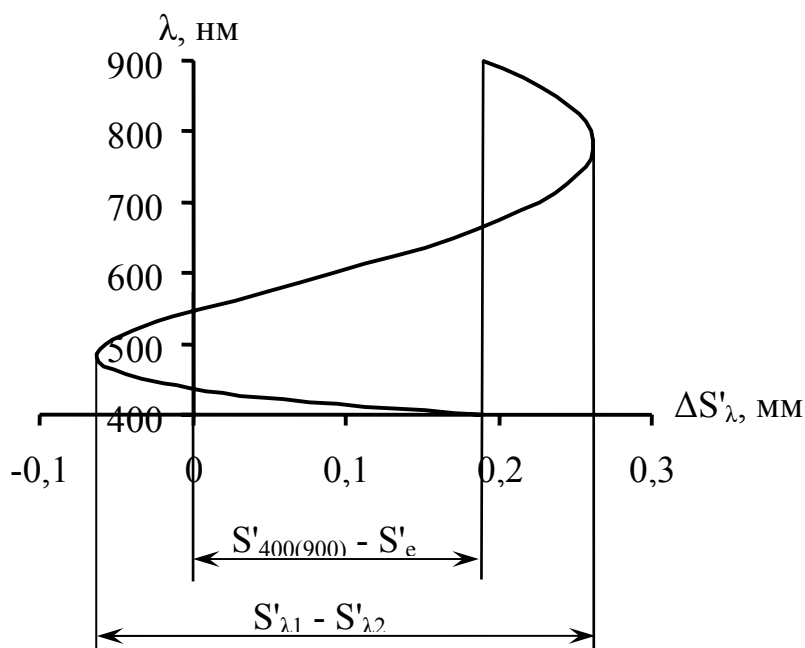
Рис.2 Вторичный спектр и остаточный хроматизм системы с f'=1000\text{мм} , выполненной из стекол ОК1 и СТК12
