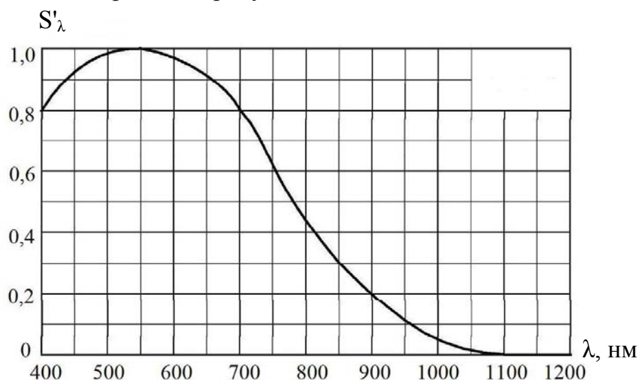
Рис.5 Спектральная чувствительность кремниевого приемника оптического излучения (TOSHIBA TCD 1304).
