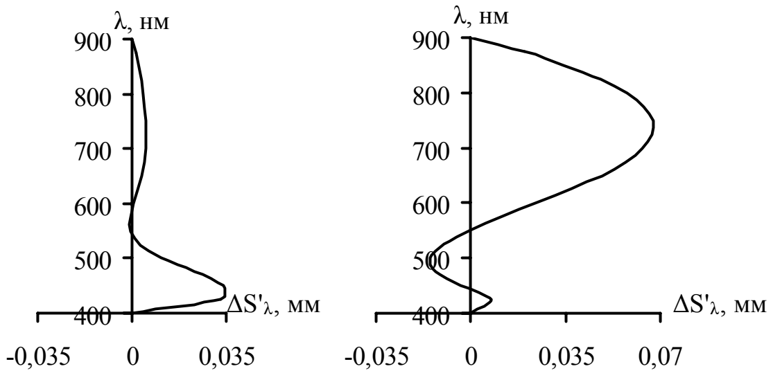
а) СТК16 – ТБΦ3 – ОК1
