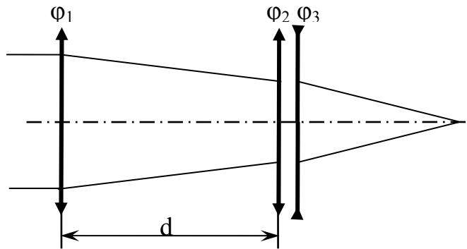
Рис.6 Схема двухкомпонентной апохроматической системы из обычных стекол: \varphi_1 – оптическая сила первого компонента, \varphi_2 – оптическая сила первой линзы второго компонента, \varphi_3 – оптическая сила второй линзы второго компонента, d – расстояние между компонентами.
