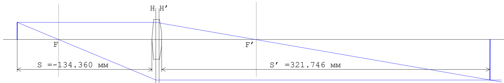
Рис.4. Построение изображения в 1-ой линзе. Масштаб 1:2.
