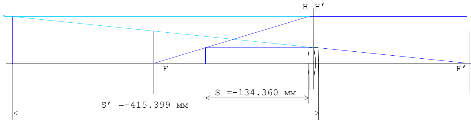
Рис.2. Построение изображения в объективе. Масштаб 1:3
