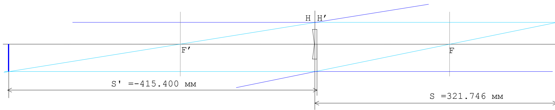
Рис.6. Построение изображения во 2-ой линзе. Масштаб 1:3.
