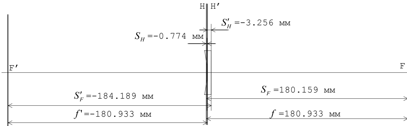
Рис.5. Кардинальные точки и отрезки 2-ой линзы. Масштаб 1:1.
