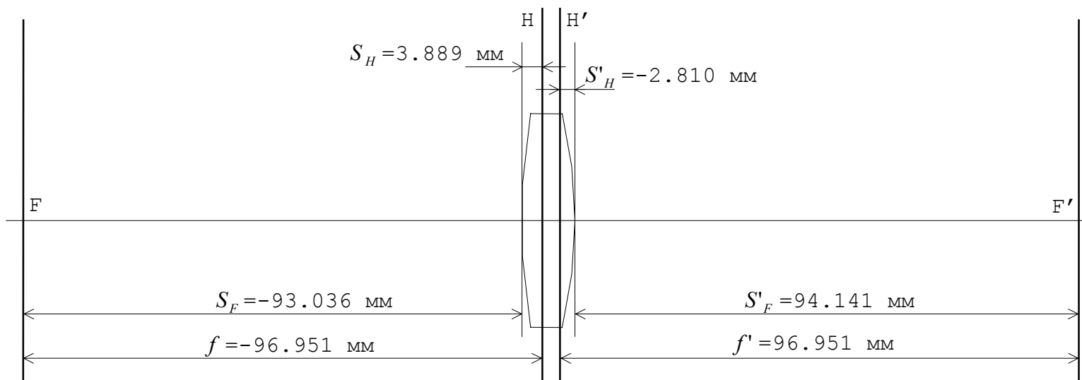
Рис.3. Кардинальные точки и отрезки 1-ой линзы. Масштаб 1:1.
