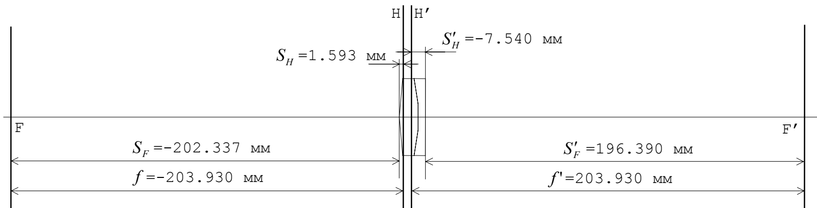
Рис.1. Кардинальные точки и отрезки объектива. Масштаб 1:2
